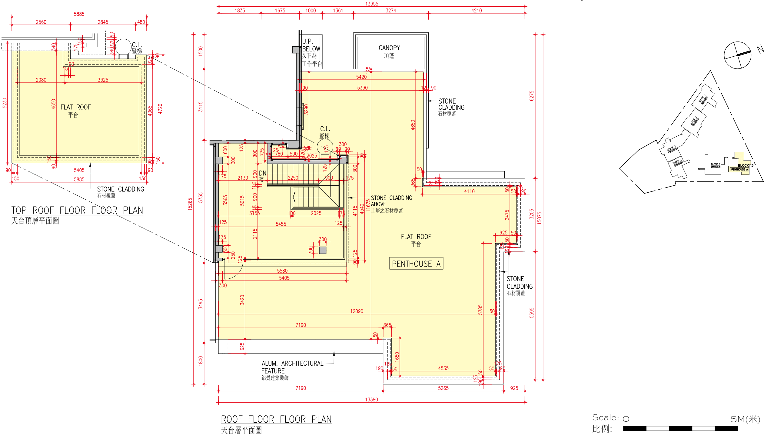
第3座 | Roof Floor & Top Roof Floor 天台層及天台頂層
