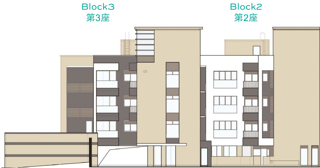
Elevation Plan F 立面圖 F
